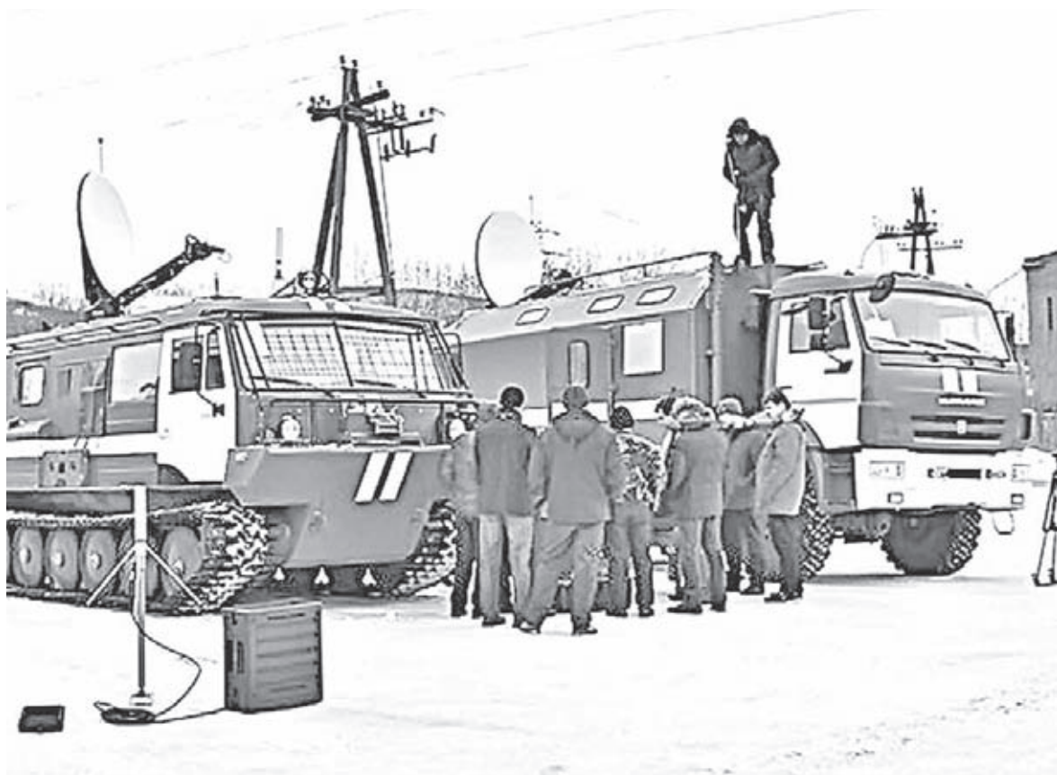
■ Самая большая проблема в тайге при тушении больших пожаров – координация мобильных групп, взаимодействие с другими ведомствами. Поэтому самые высокие требования предъявляются к связи – от нее в тайге зависит жизнь. Фото краевого лесопожарного центра
